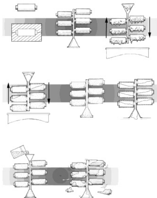
Figuur 7.1 Schematisch overzicht verloren wasgieten
